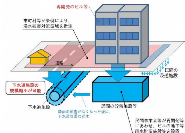
官民連携による浸水被害対策として、民間の貯留施設等の設置や浸透施設の設置を促す制度等の活用（官民連携した浸水対策の手引き（案））
