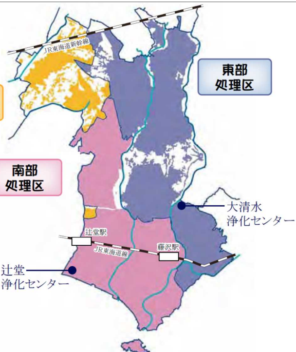
図 5-11 公共下水道整備計画区域
